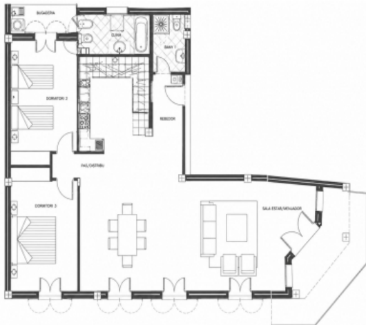
Grundriss
