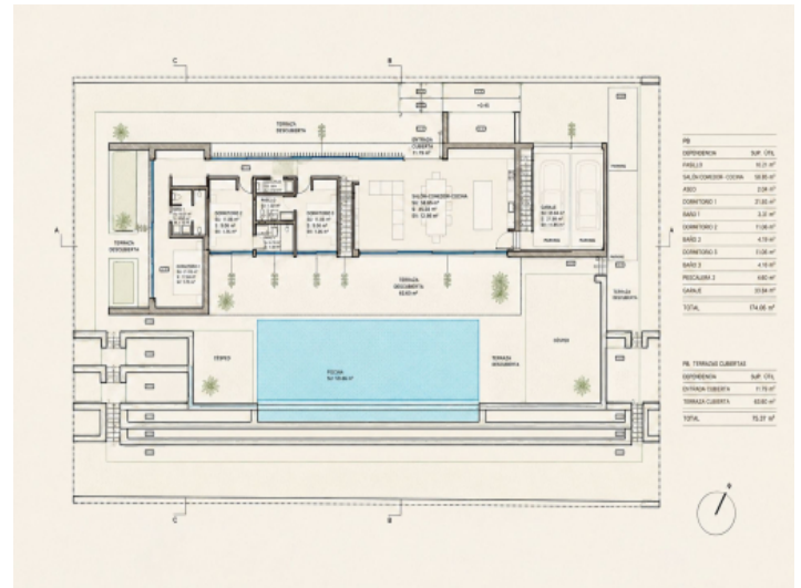
Grundriss Wohnebene
