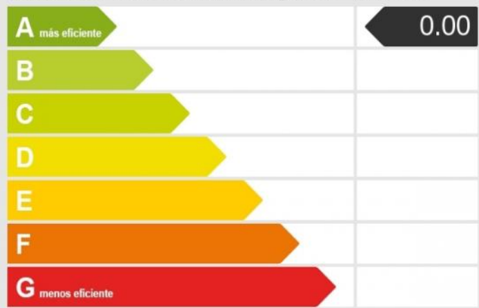
Energieskala
