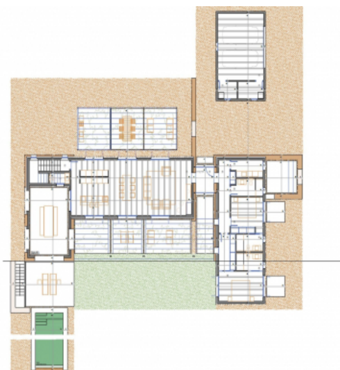
Grundriss Erdgeschoss
