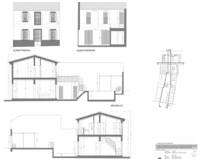
Bauplan
