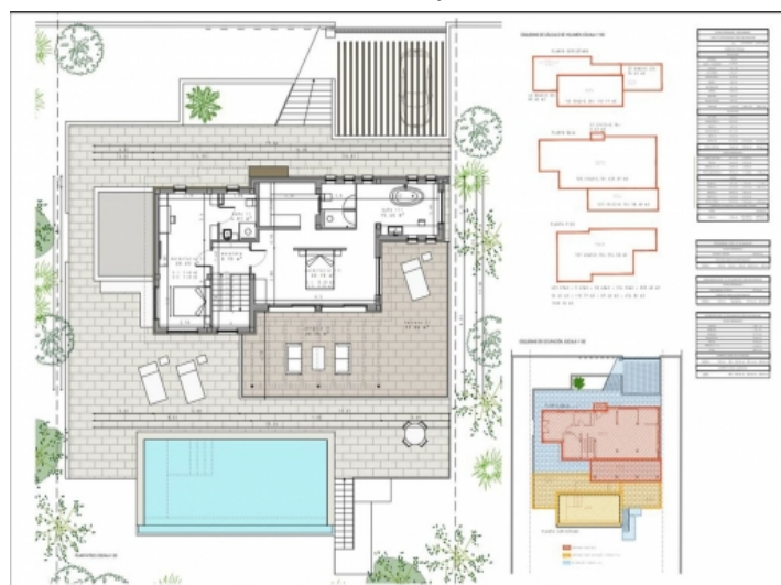
Erste Etage
